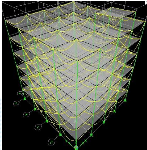
تغییر شکل سازه تحت بار مرده
